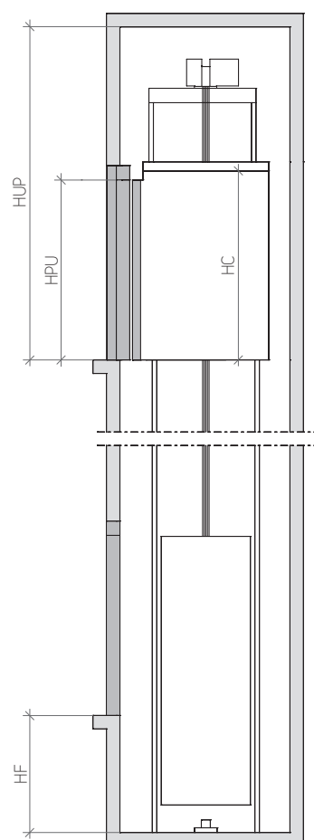
SEZIONE VERTICALE
